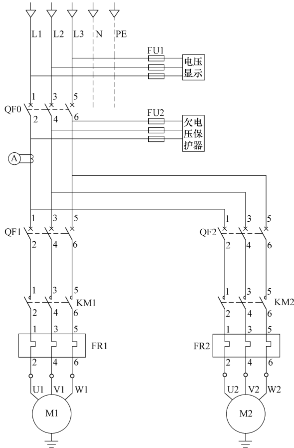
图 1-11 电路图示例
