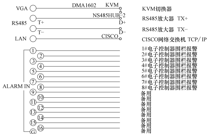
图 1-19 接线图示例
