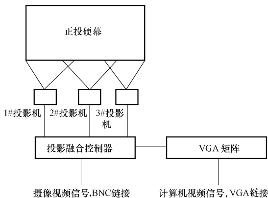
图 1-16 安装简图示例
