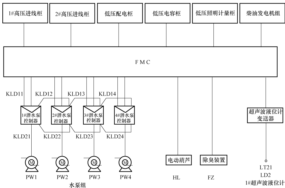
图 1-5 FMC 控制功能图
