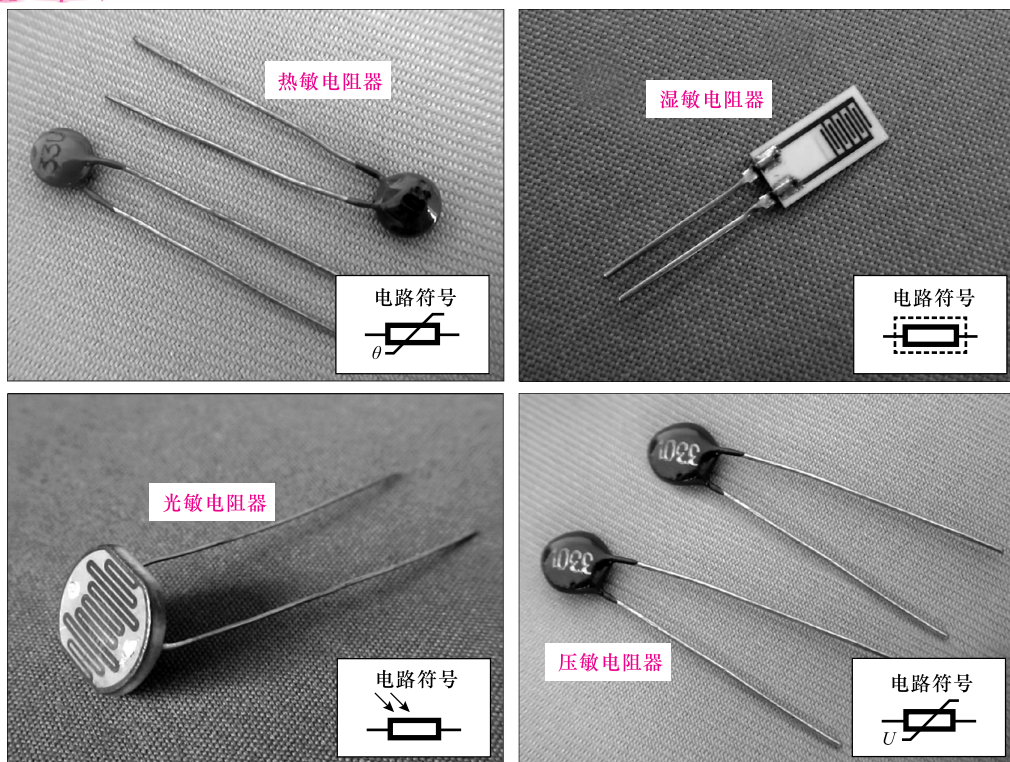
图 1-4 敏感电阻器的实物外形
