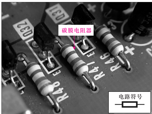
图 1-1 薄膜电阻器的实物外形
