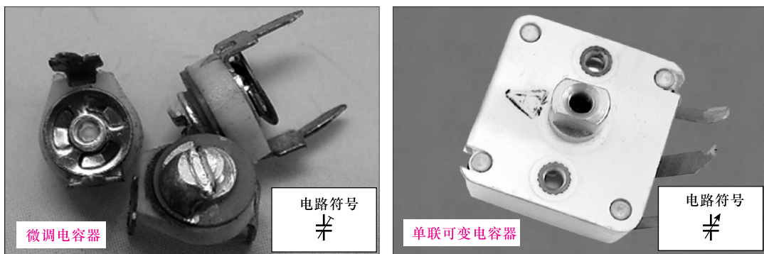
图 1-13 可变电容器的实物外形
