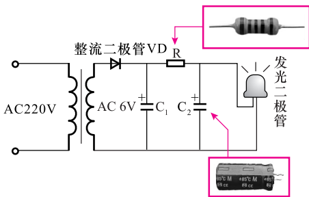
图 1-9 电阻器的滤波作用
