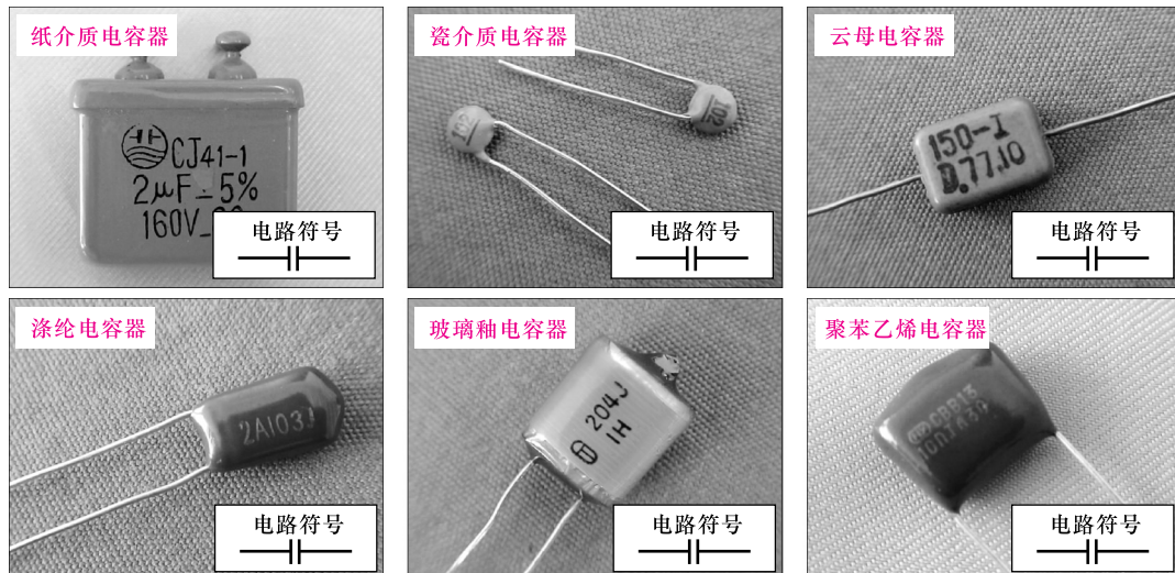
图 1-10 无极性固定电容器的实物外形
