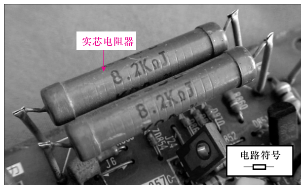
图 1-2 实芯电阻器的实物外形
