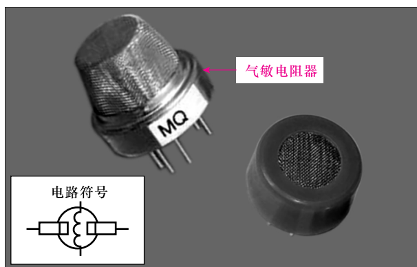
图 1-5 气敏电阻器的实物外形
