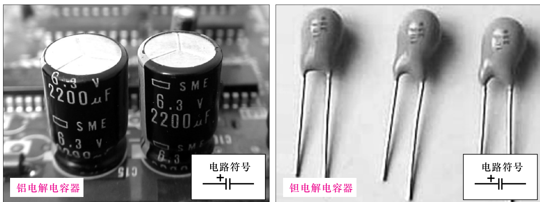
图 1-12 有极性固定电容器的实物外形
