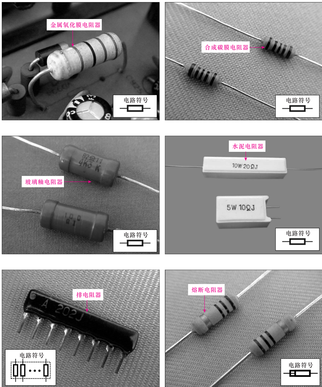
图 1-1 薄膜电阻器的实物外形 (续)
