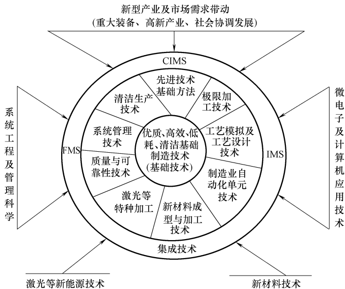
图 1-1 AMST 的多层次先进制造技术体系结构
