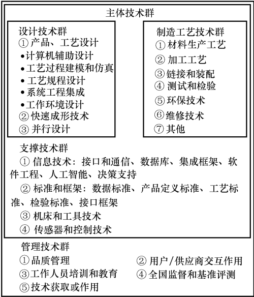
图 1-2 FCCSET 的先进制造技术体系结构
