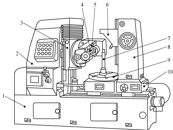
图 1-9 Y3150E 型滚齿机
