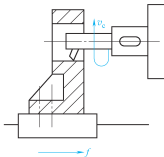
图 1-6 镗削加工
