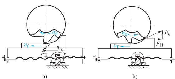
图 1-3 顺铣和逆铣
