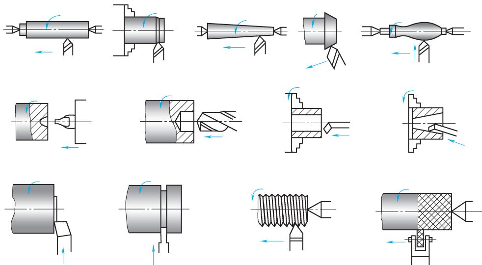
图 1-1 车床加工的典型工序
