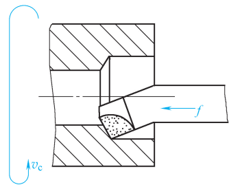
图 1-7 车床镗孔
