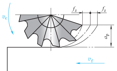
图 1-2 铣削加工
