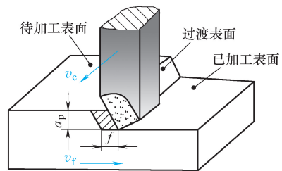
图 1-4 刨削加工
