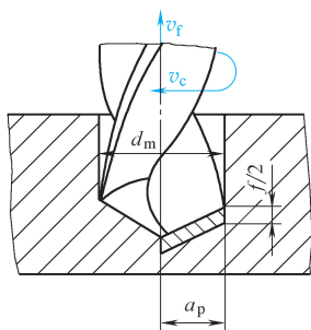
图 1-5 钻削加工
