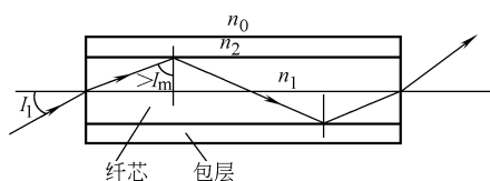
图 1-6 光纤的基本结构和全反射传光原理
