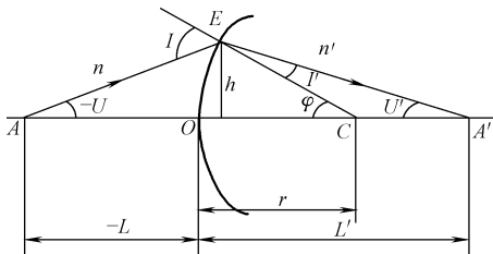
图 1-11 光线经过单个折射球面的折射
