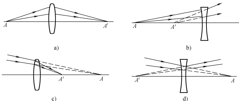
图 1-10 物、像的虚实
