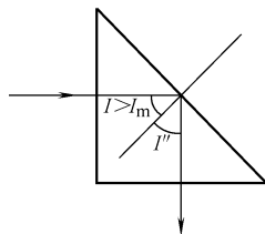
图 1-5 全反射直角棱镜
