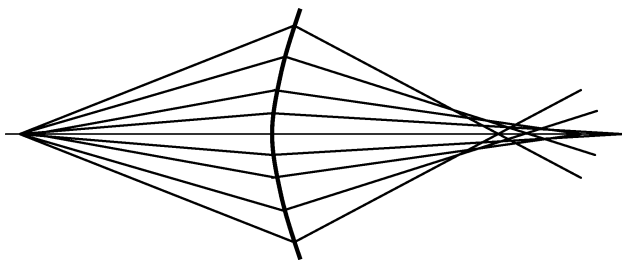
图 1-12 轴上点成像的不完善性
