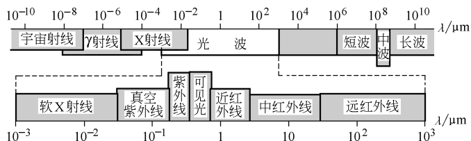
图 1-1 电磁波谱
