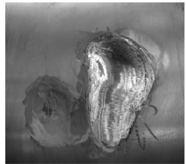
图 3 打磨后剥落处形态
