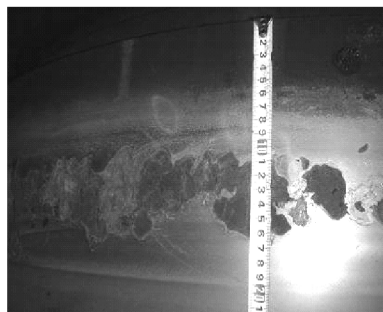
图2 辊面剥落掉肉
