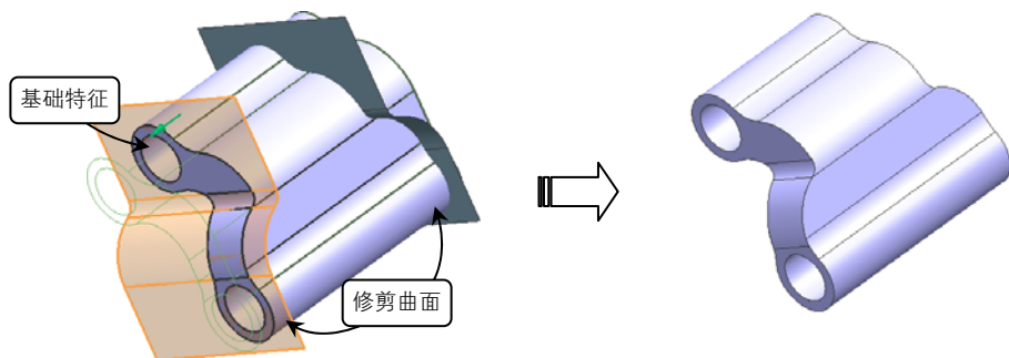
图 1-12 修剪法创建实体
