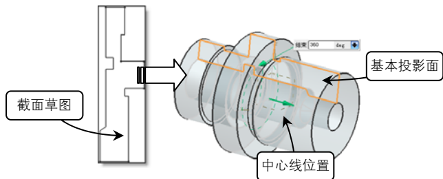
图 1-3 回转体截面生成实体
