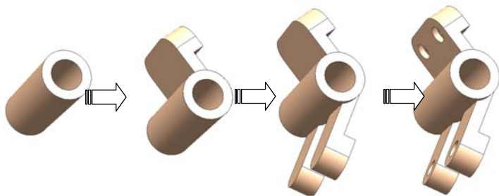
图 1-10 积木法创建三维实体
