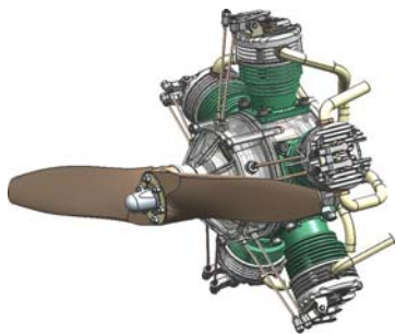
图 1-3 飞机引擎装配体
