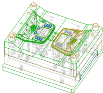
图 1-4 电子设备外壳模具机构
