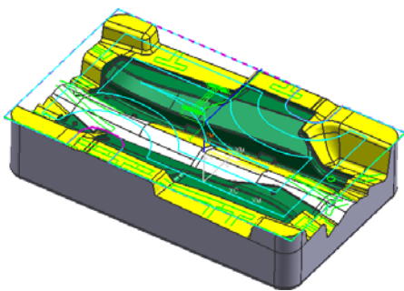
图 1-5 型腔铣削刀路
