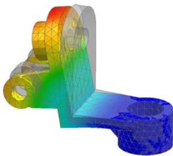
图 1-6 支座有限元分析
