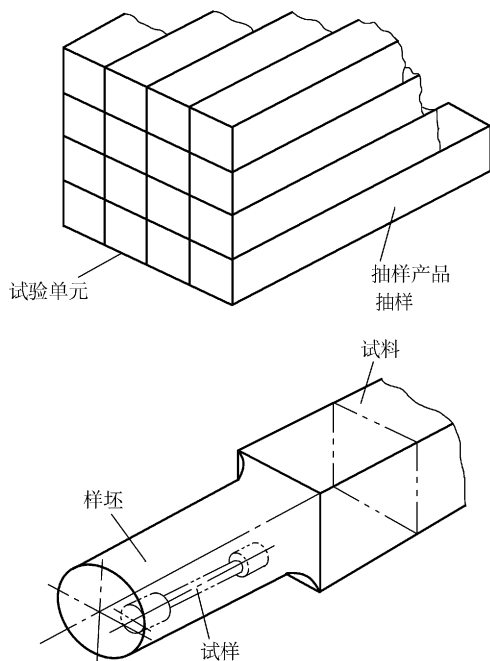
图 1-1 试验单元、抽样产品、试料、样坯及试样
