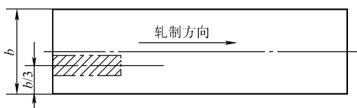
图 1-5 扁钢取样部位
