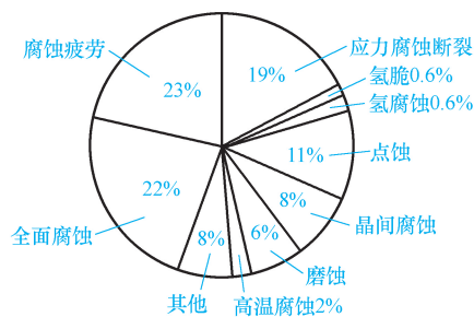
图0-2 金属各种腐蚀形态的比例
