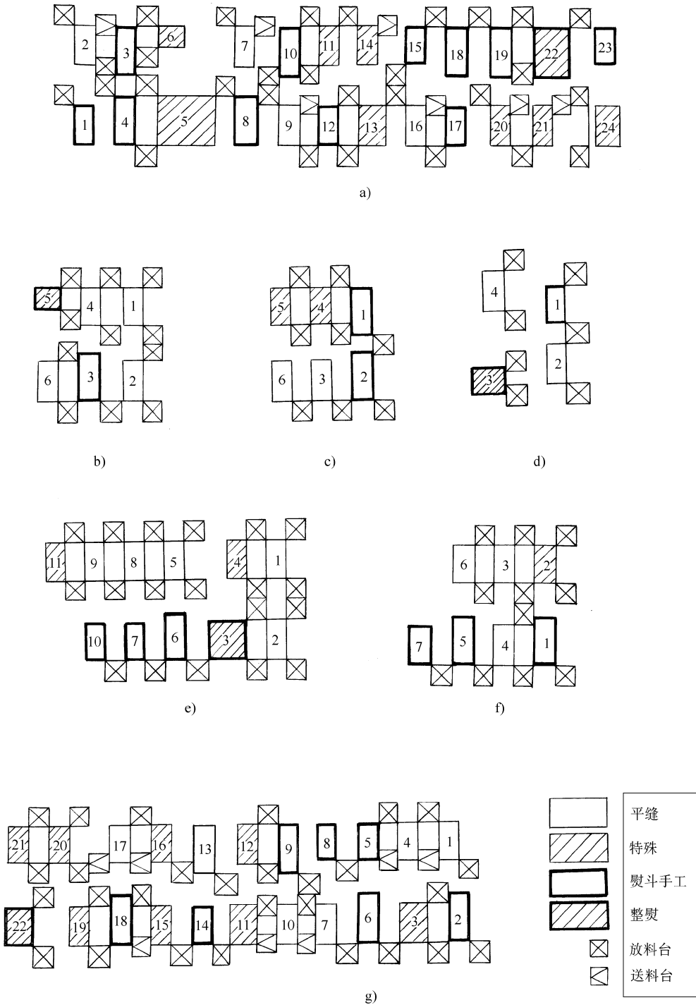
图 1-2 西服生产线设备排列
