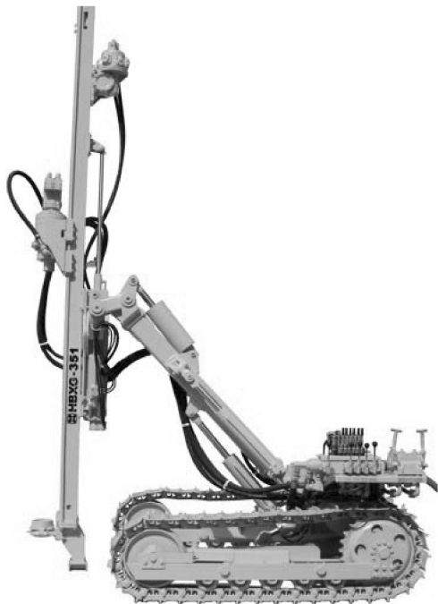
图 1-1 履带式底盘
