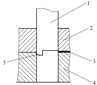
图 1-2 防倾侧结构 1—凸模 2—卸料板 3—制件 4—凹模 5—凸模导向部分
