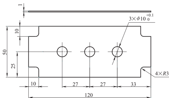
图 1-1 连接板
