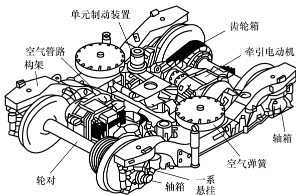
图 1-1 动车转向架
