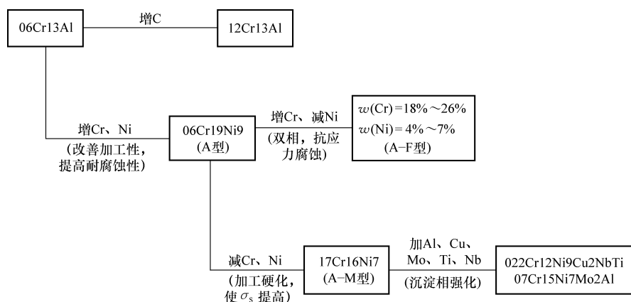
图 1-1 各类不锈钢成分之间的关系
