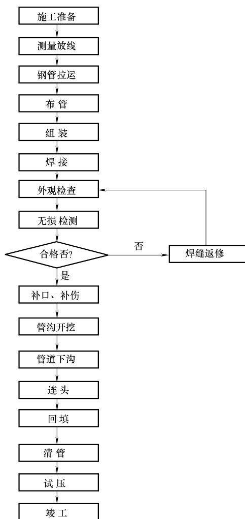
图 1-2 长输管道施工工艺流程
