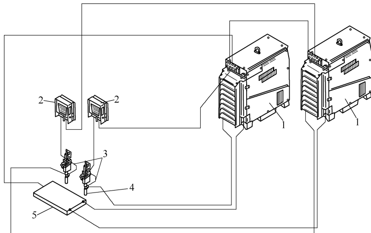
图 1-15 双丝串联埋弧焊机头与焊接电源及控制器之间的连接方式
