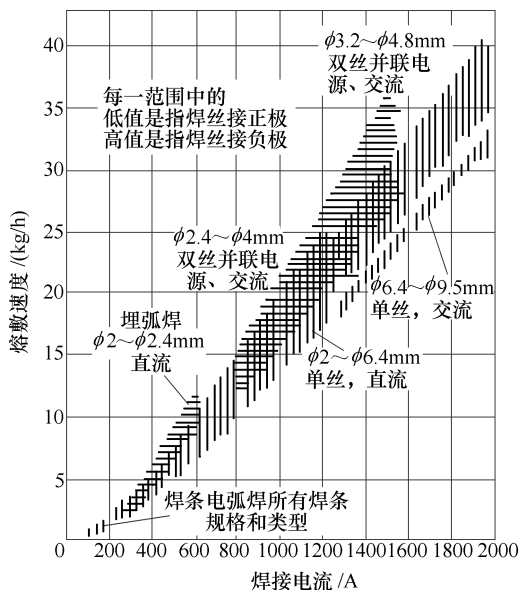
图 1-3 各种埋弧焊方法与焊条电弧焊熔敷速度的对比
