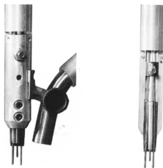
图 1-26 集束冷丝埋弧焊导电嘴的结构外形
