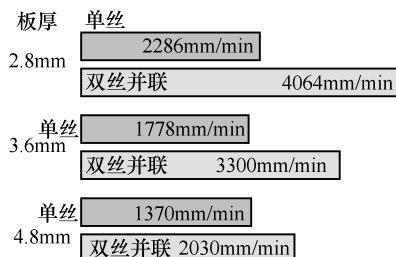
图 1-13 搭接接头焊接速度对比
