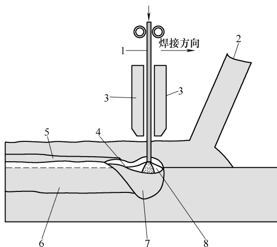
图 1-1 埋弧焊过程原理图
