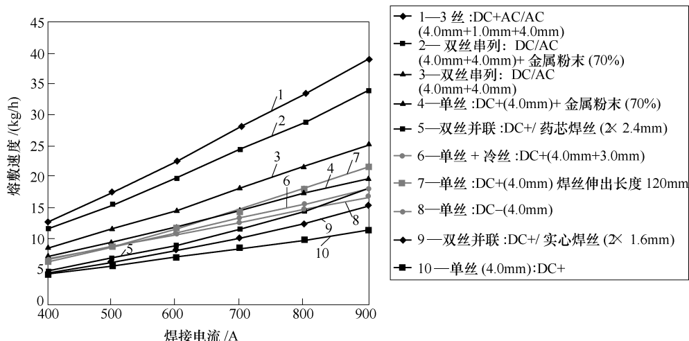
图 1-18 三丝埋弧焊与其他各种埋弧焊熔敷速度的对比
