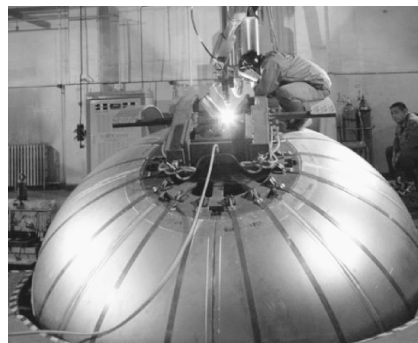
图 1-13 贮箱箱底焊铣复合加工系统
