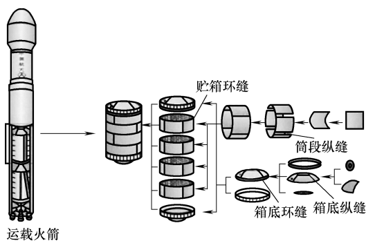
图 1-9 运载火箭贮箱结构示意图
