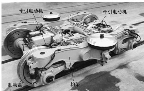
图 1-24 动车转向架
