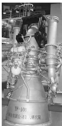
图 1-15 YF-100 发动机
