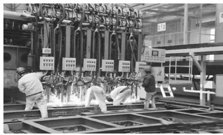
图 1-31 肋板焊接
