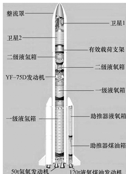
图 1-8 火箭结构示意图
