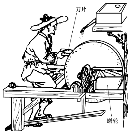
图 0-6 古代脚踏刃磨机
