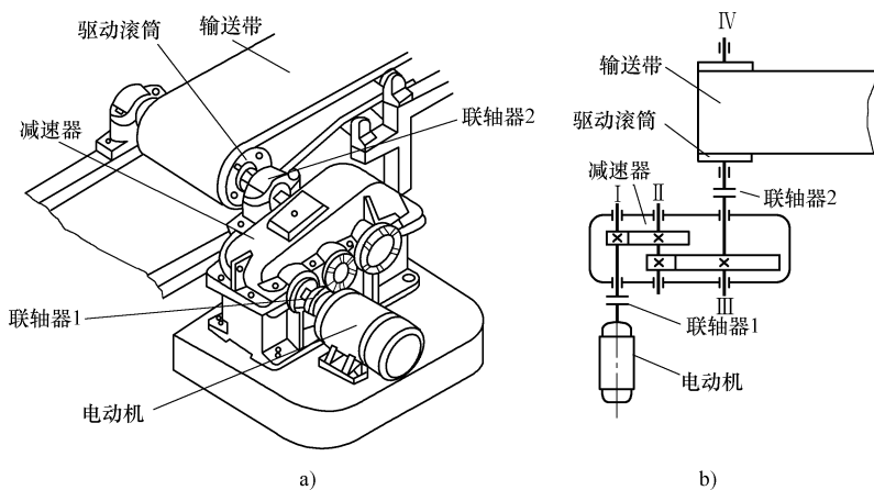
图 1-1 带式输送机传动装置
