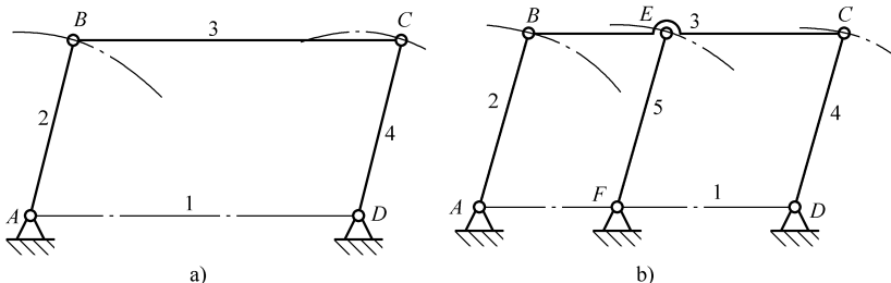
图 1-9 虚约束
