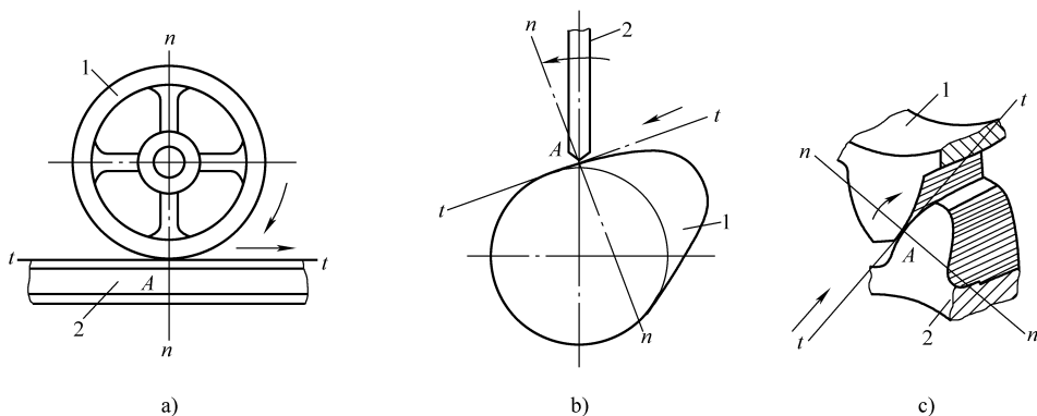
图 1-4 平面高副
