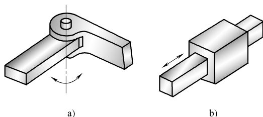
图 2-2 平面低副 a) 转动副 b) 移动副
