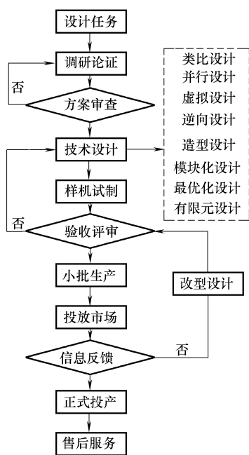
图 1-3 机械设计制造的一般程序框图
