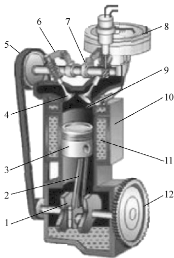
图1-2 单缸内燃机
