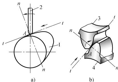
图 2-3 平面高副 a) 凸轮副 b) 齿轮副 1—凸轮 2—从动件 3、4—轮齿
