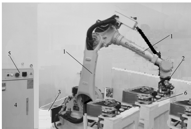
图 1-1 专用装配机器人
