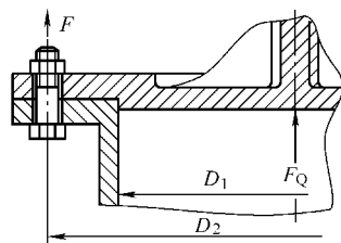
图 1-1 螺栓组连接受轴向载荷作用
