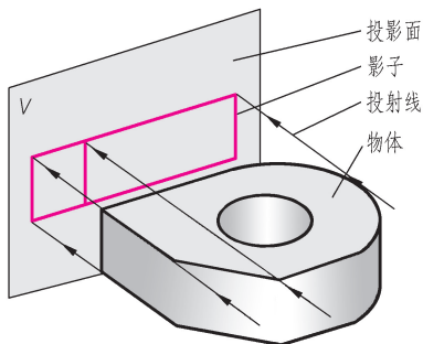
图 1-1 影子的产生
