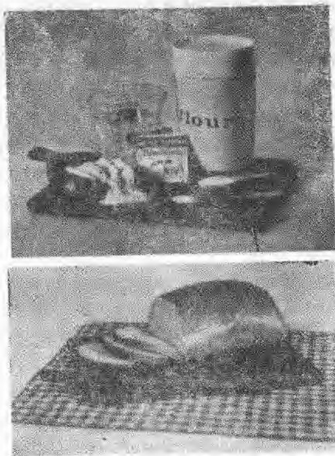
图 1-2 化学变化。一块面包的组成成分不同于烘烤前的液体或固体混合物的成分。在烘炉里,糖、面粉和盐进行了许多化学变化。烘烤前,化学变化是由酵母释放二氧化碳引起的,二氧化碳使面包发起来。没有一种物理性质能够使面包恢复到它的先前成分。(当你看到面包,而不是看到面包的成分时,你的嘴可能会变得湿润。这表明你的身体对食物的条件反射,准备在体内进行化学变化。)
