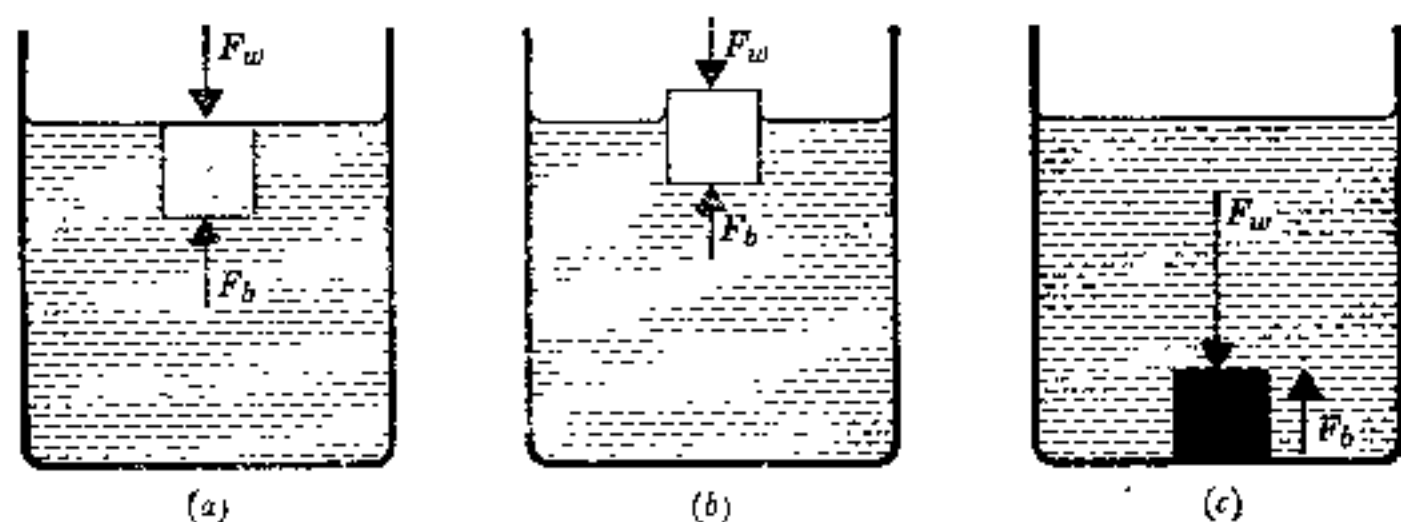
图 1-3 阿基米德原理。(a)、(b)、(c)中的立方体体积相同,但是由于组成材料不同,因而密度各不相同。由于(b)中的立方体密度最小,所以它最轻。(c)中的立方体密度最大,所以它最重。(a)中的立方体居中,它的重力 F_w ,正好等于相应体积液体的重量。当立方体下沉到所示的位置时,所产生的浮力 F_b 等于 F_w 。(b)图为了使产生的浮力等于这个较轻的立方体的重量,只须排出少量液体。因此,立方体只是部分浸在水中。(c)图中,被排出液体的重量,即所产生的浮力不足以支撑较重的立方体,因此这个立方体就沉到底部。
