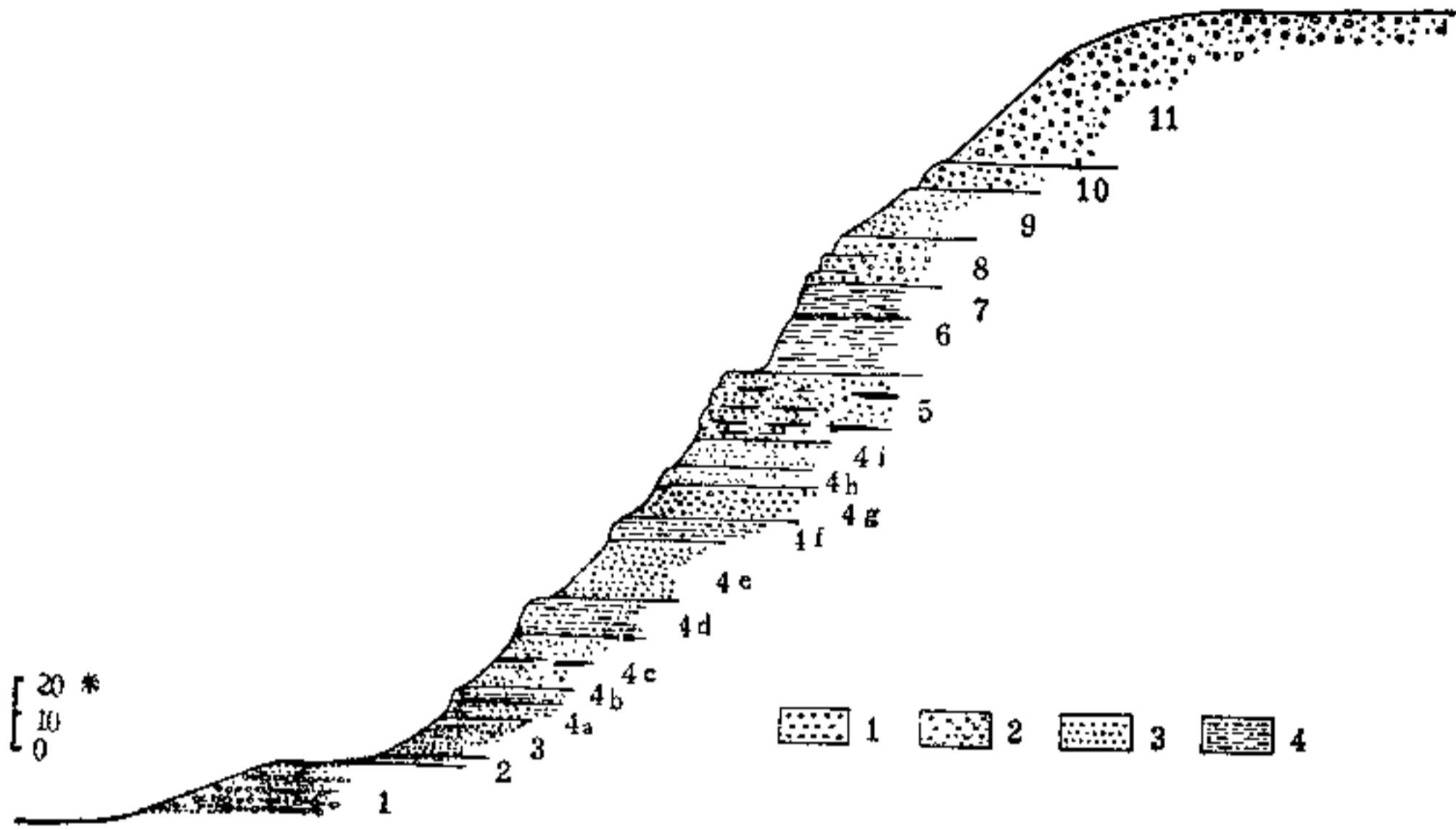
1 砾岩 2 砂砾岩 3 砂岩 4 砂质粘土岩
