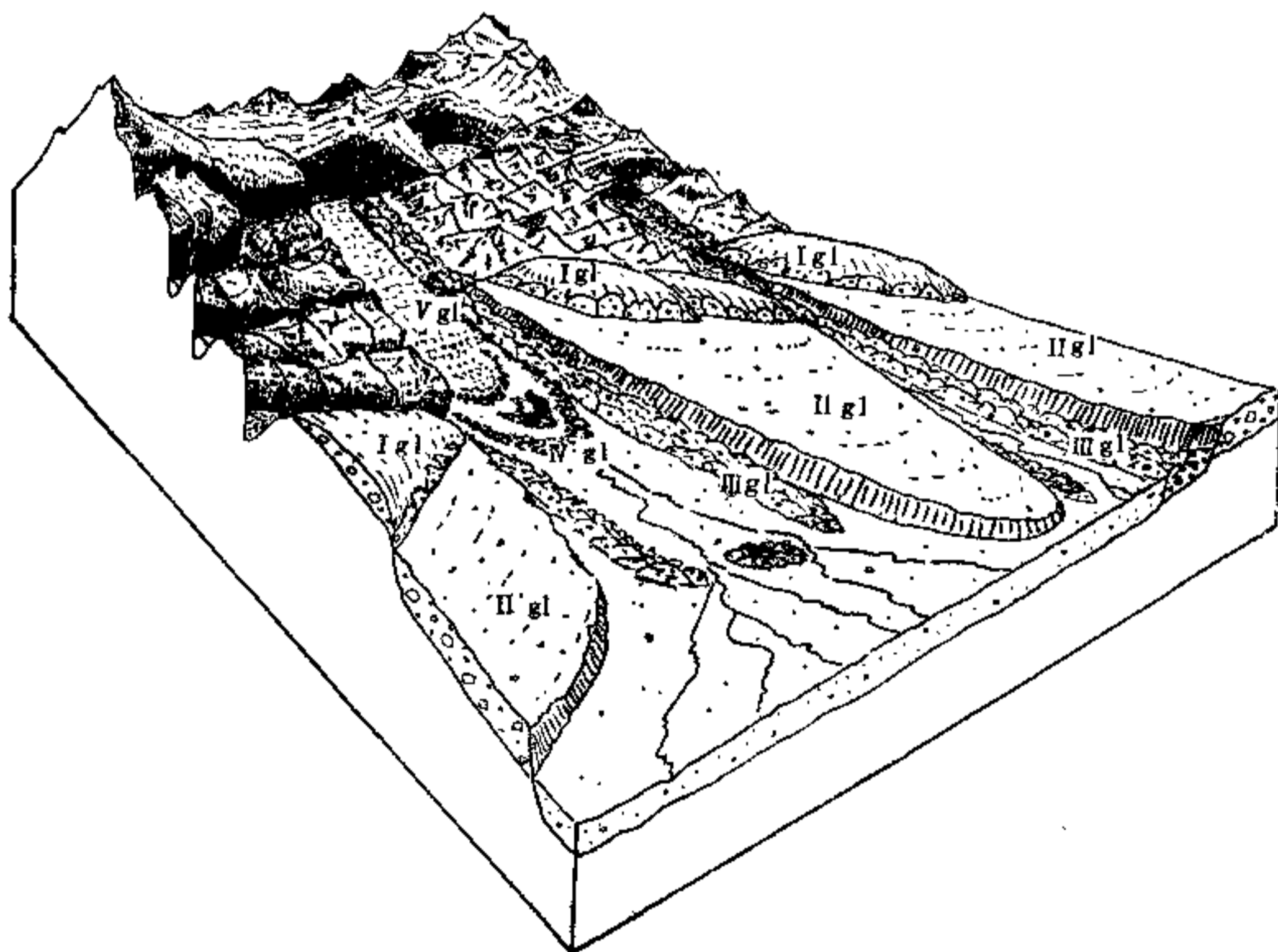
Igl, 希夏邦马冰期冰碛; IIgl, 聂聂雄拉冰期冰碛; IIIgl, 珠穆朗玛冰期冰碛; IVgl, 绒布德小冰期冰碛; Vgl, 现代冰川。
