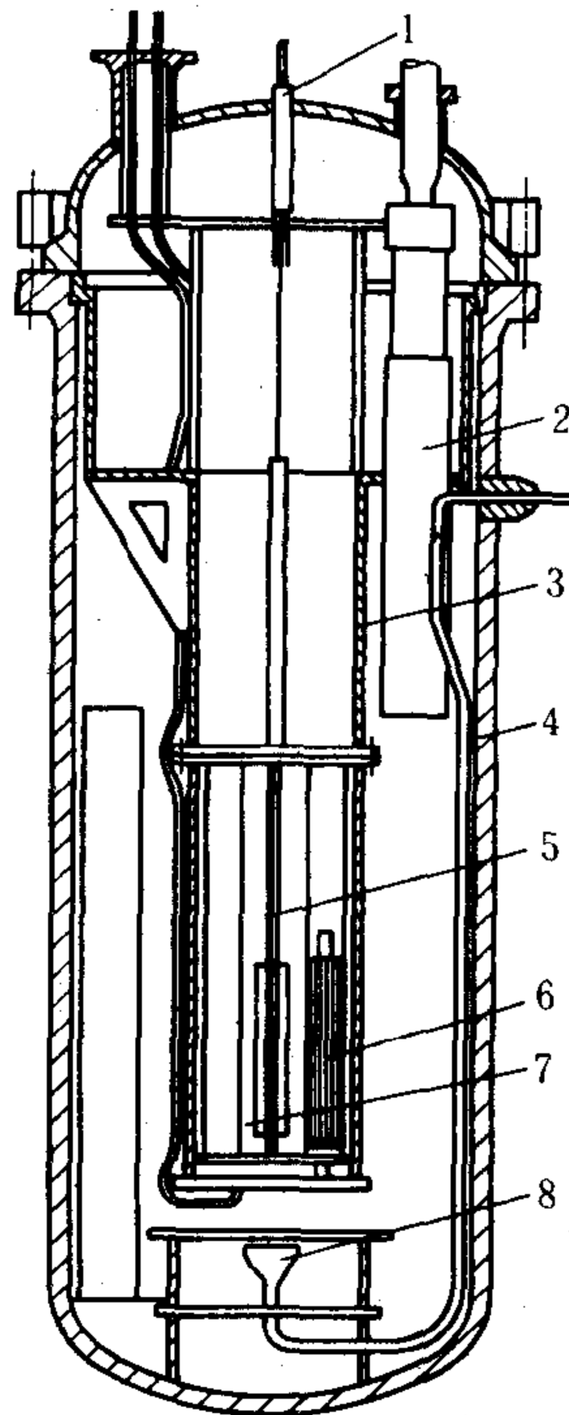
图 1 5兆瓦核供热堆布置示意图
