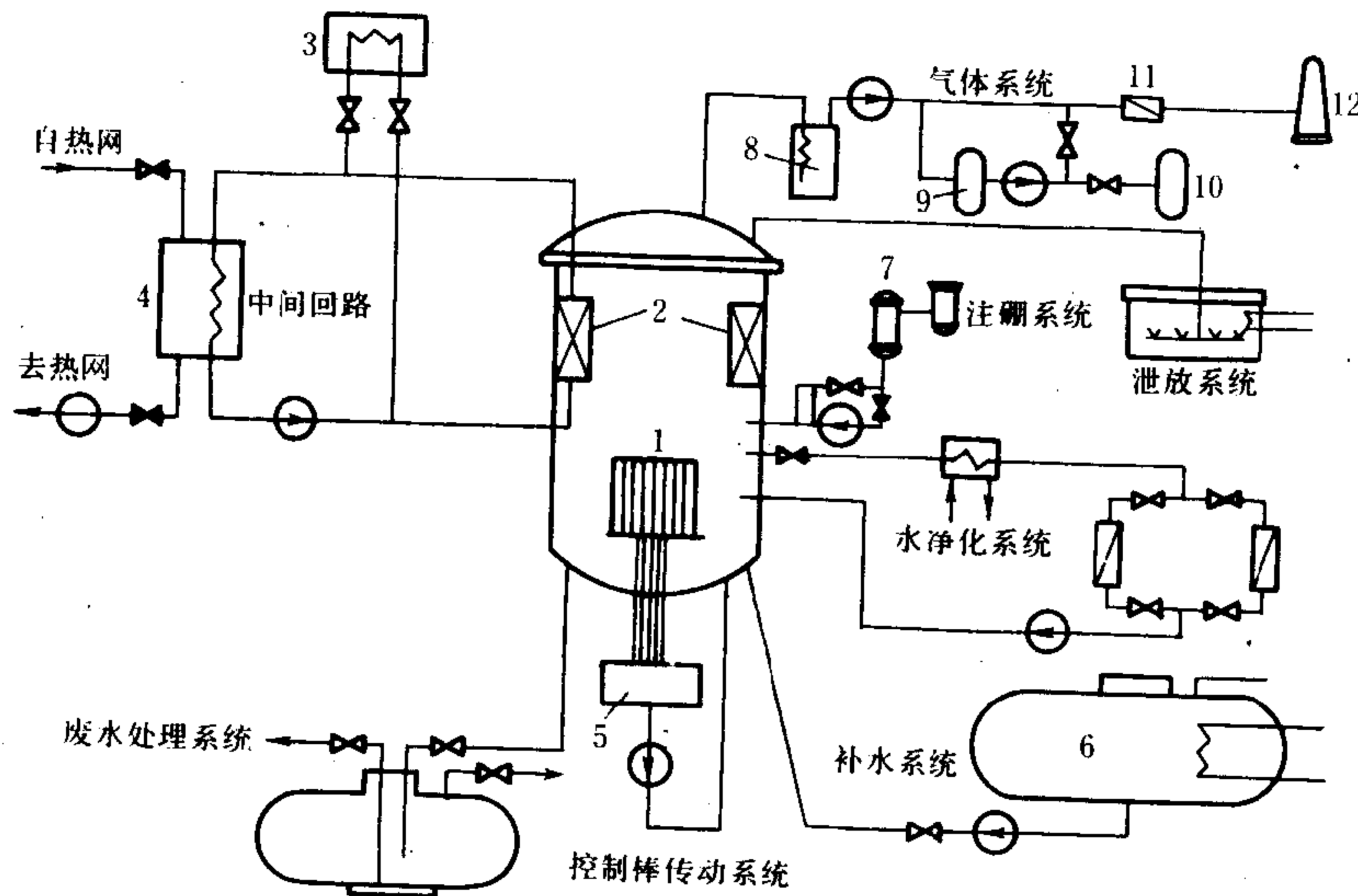
图2 5兆瓦供热堆系统示意图
