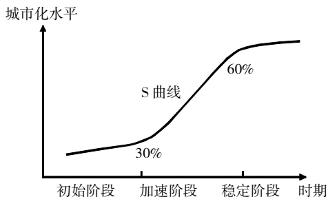
图 1-1 诺瑟姆曲线(城市化过程曲线)
