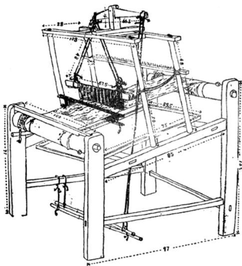
◎图1-9 缂丝机
