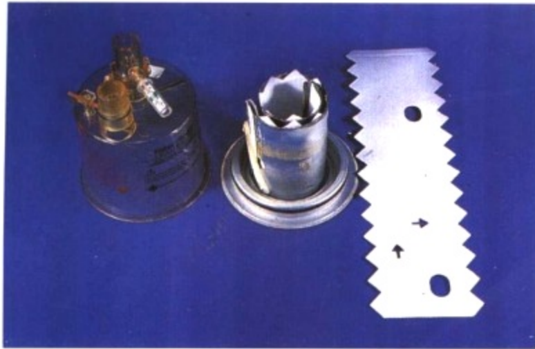
(b) 改良式内部结构
