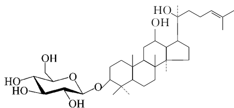
人参皂苷 Rh 2
