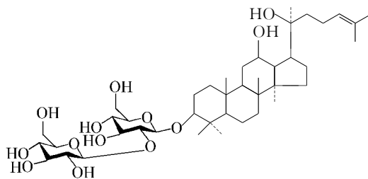
人参皂苷 Rg_3
