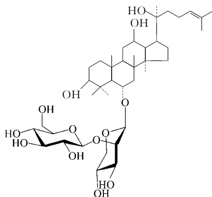
人参皂苷 Rg 2
