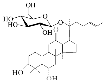
人参皂苷 Rh 8
