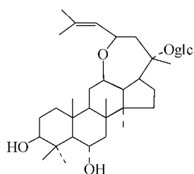
人参皂苷 Rh 9
