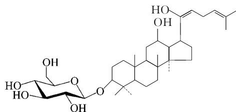
人参皂苷 Rh_3
