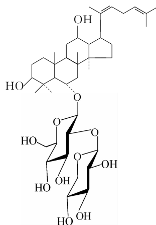
20( E )-人参皂苷 F_4
