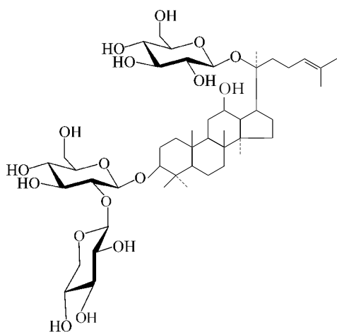
三七参苷 R_1
