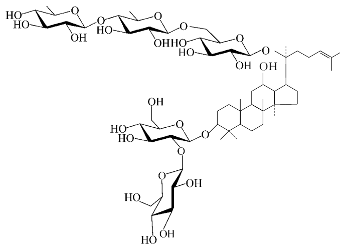
人参皂苷 Ra 1
