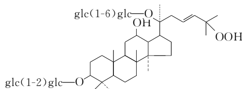
三七参苷 E
