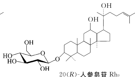
20( R )-人参皂苷 Rh_2
