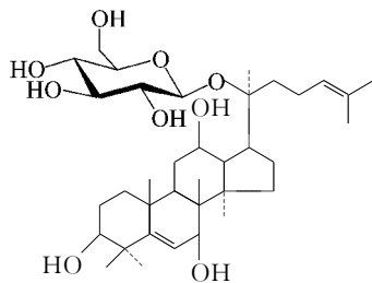
人参皂苷 Rh 7
