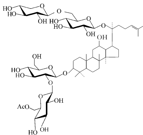
人参皂苷 Rs_1
