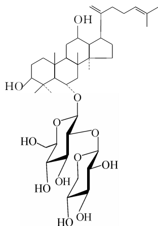
人参皂苷 Rg_6
