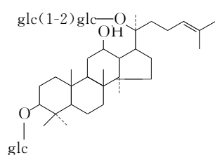
绞股蓝皂苷 XVII
