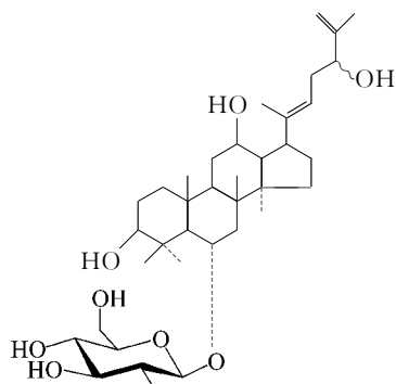
人参皂苷 Rh 5
