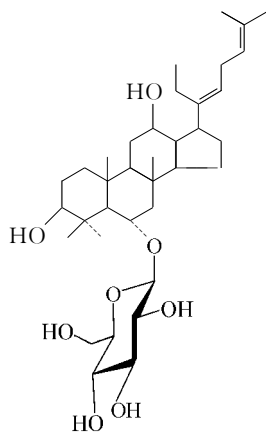
人参皂苷 Rh 4
