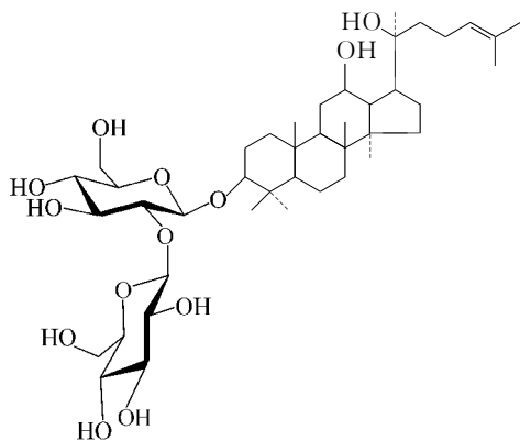
20(S)-人参皂苷 Rg 3
