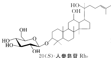
20( S )-人参皂苷 Rh_2
