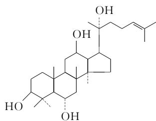
20( R )-原人参三醇
