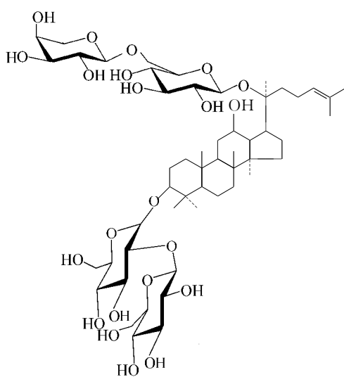
人参皂苷 Rb 2
