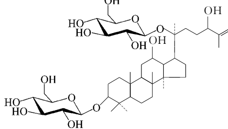
人参皂苷 Rg 7
