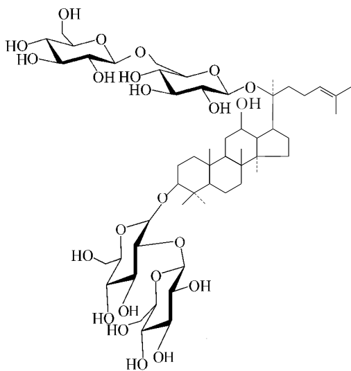
人参皂苷 Rb 1
