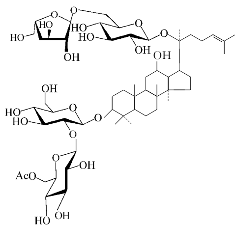
人参皂苷 Rs_2
