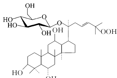
人参皂苷 Rh 6
