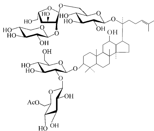
人参皂苷 Ra_2
