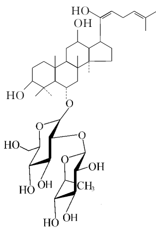
人参皂苷 F_4
