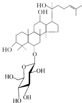
人参皂苷 Rh_1
