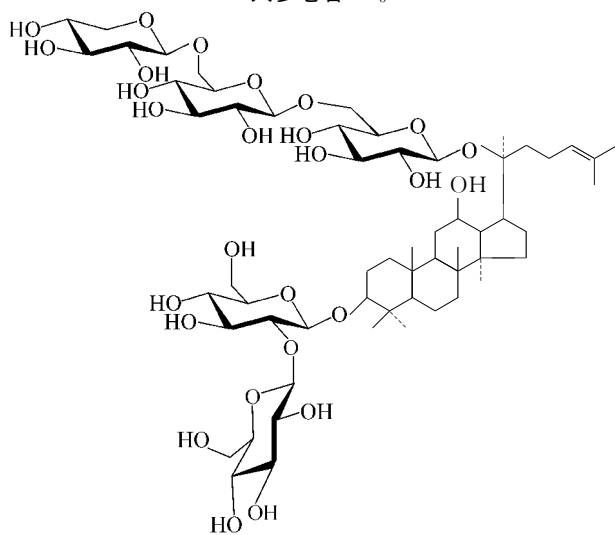
三七参苷 R_4
