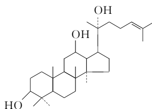
20( R )-原人参二醇
