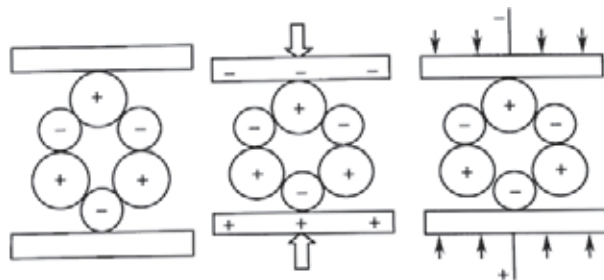
图 1-1-1 压电效应原理示意图
