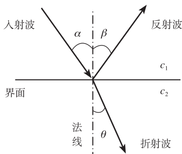
图 1-2-1 超声的反射与折射
