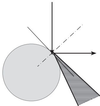
图 1-2-5 超声全反射声影形成示意图
