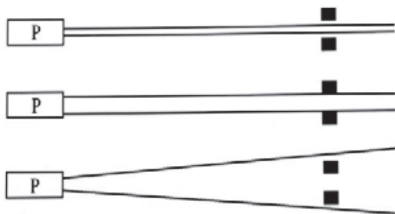
图 1-2-9 不同声束宽度对侧向分辨力影响示意图
