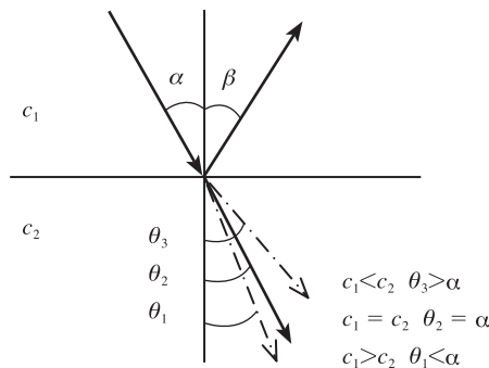
图 1-2-3 不同介质中声束折射规律
