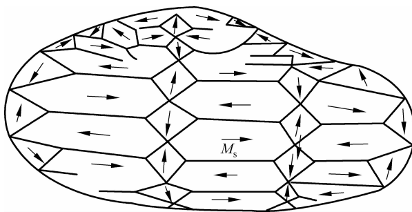
图 1-1-2 铁磁性物质内部自发磁化按磁畴的分布
