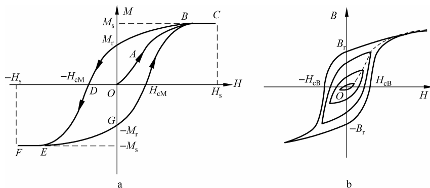
图 1-1-5 (a) 铁磁材料静态磁化的 M-H 磁滞回线; (b) 铁磁材料静态磁化的 B-H 磁滞回线
