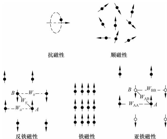
图 1-1-1 五种磁性的原子磁矩微观排列
