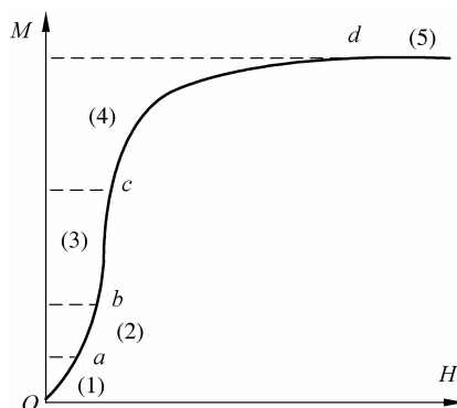
图 1-1-3 典型的铁磁材料磁化曲线
