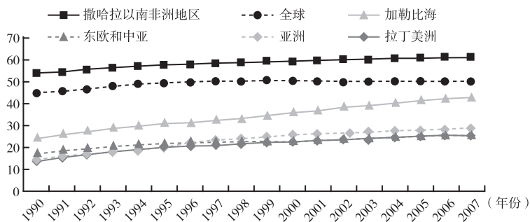
图 1-3 15 岁以上艾滋病感染者/病人中女性的比例 (1990 ~ 2007)
