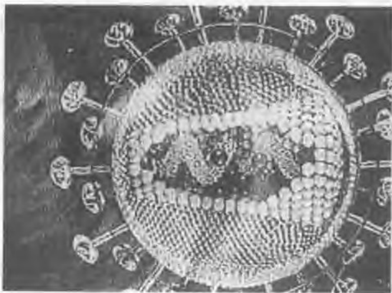
导致“非典”的新型冠状病毒
