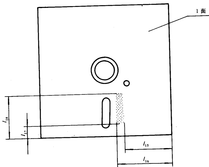
图 8 压垫区
