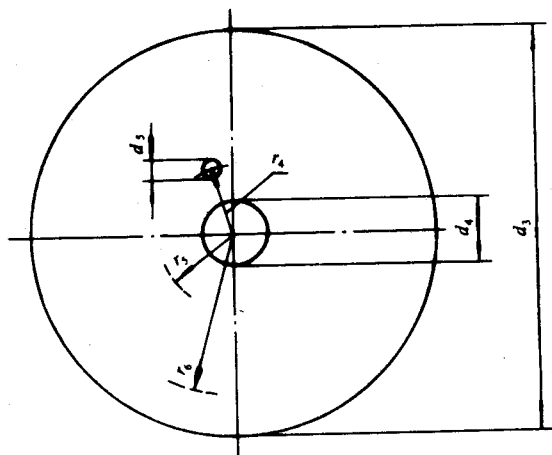
图 6 磁盘尺寸
