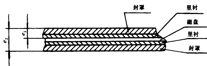
图 5 软磁盘厚度
