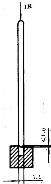
图 A2 测量量规
