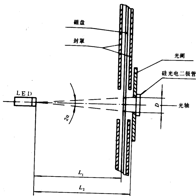
图 B1 测量装置
