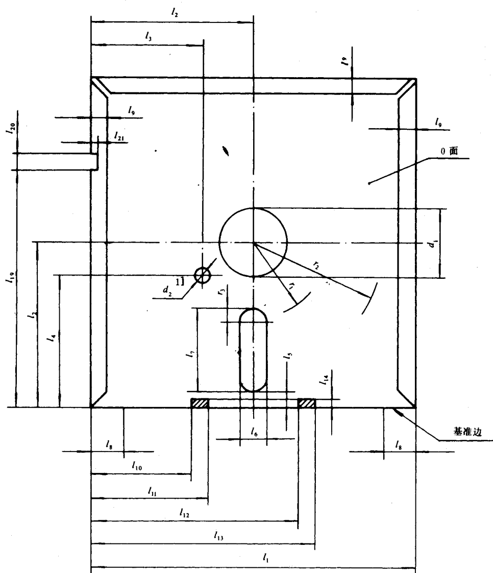
图 4 封罩尺寸 1)
