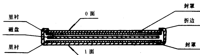
图 2 A—A 剖面图
