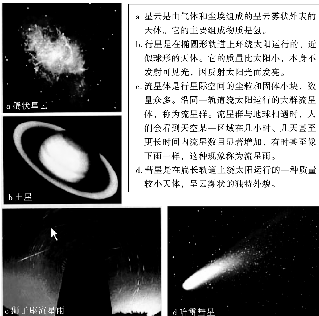
图 1-2 宇宙是由物质组成的
