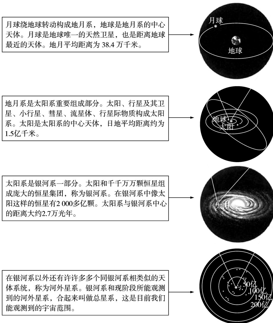
图 1-3 宇宙中不同级别的天体系统
