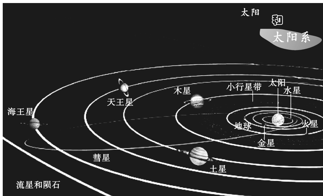
图 1-11 太阳系模式图
