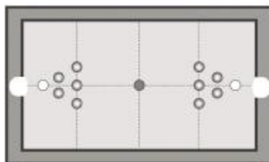
图 1-1-3 b 西安掷球台台面图
