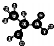
丙氨酸分子结构模型
