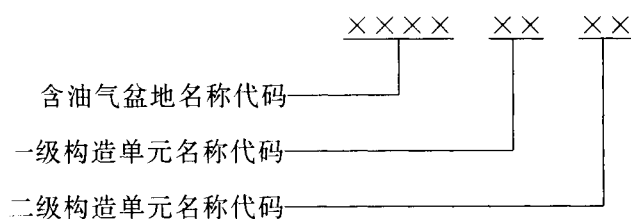
图 1 代码结构
