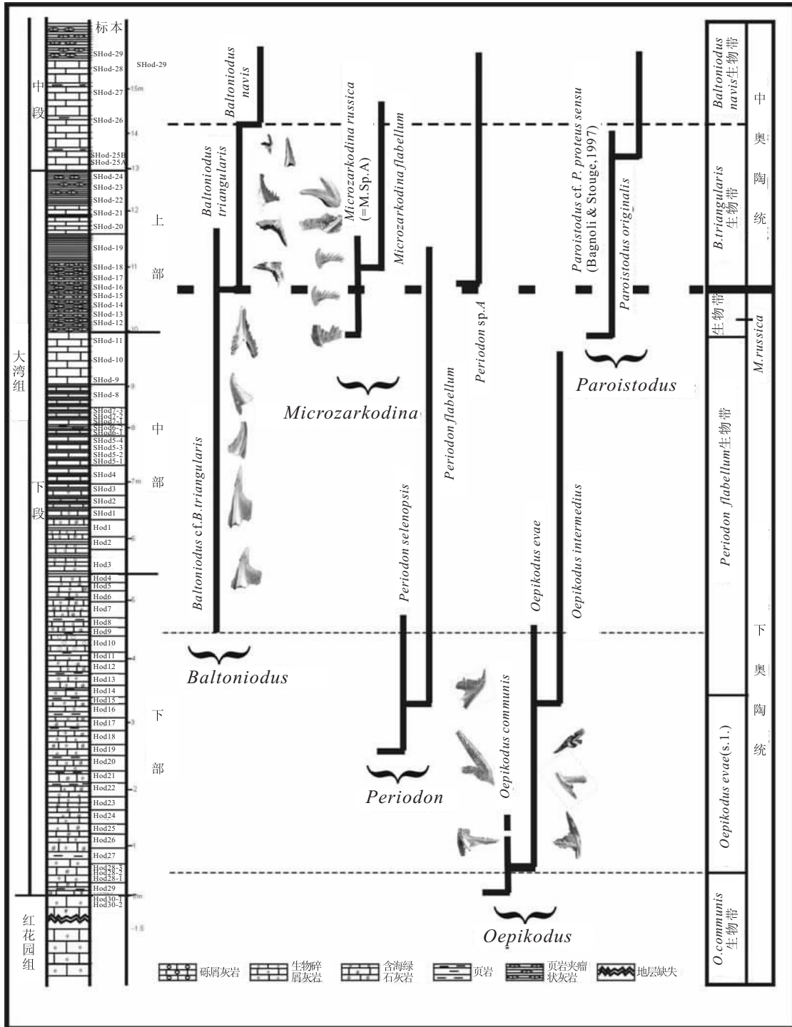
图1 黄花场剖面中奥陶统与下奥陶统界线上下牙形石谱系演化序列
