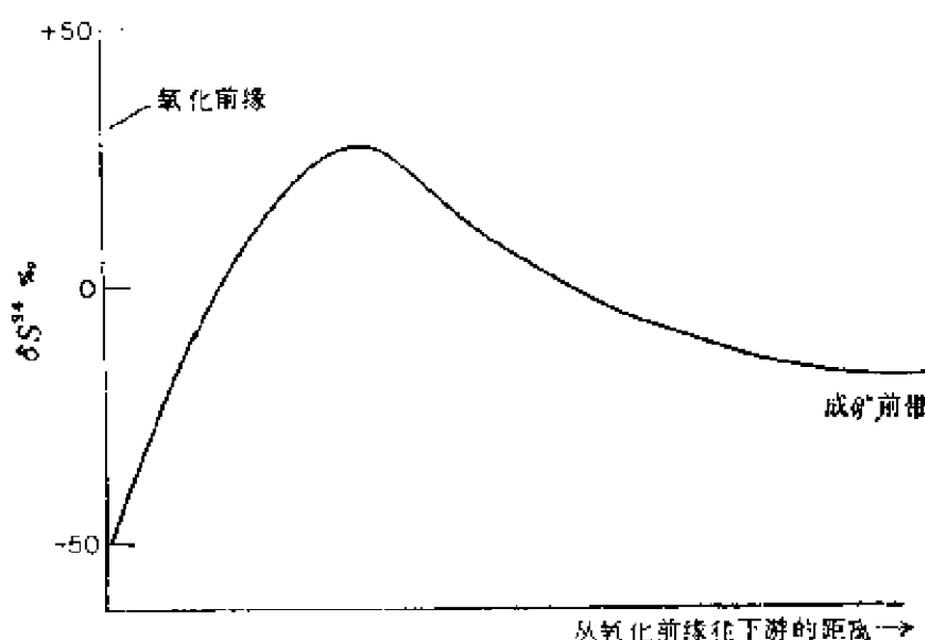
图 3 硫酸盐完全转变成黄铁矿的生物作用，整个黄铁矿的同位素含量对氧化前缘往下游的距离作图
