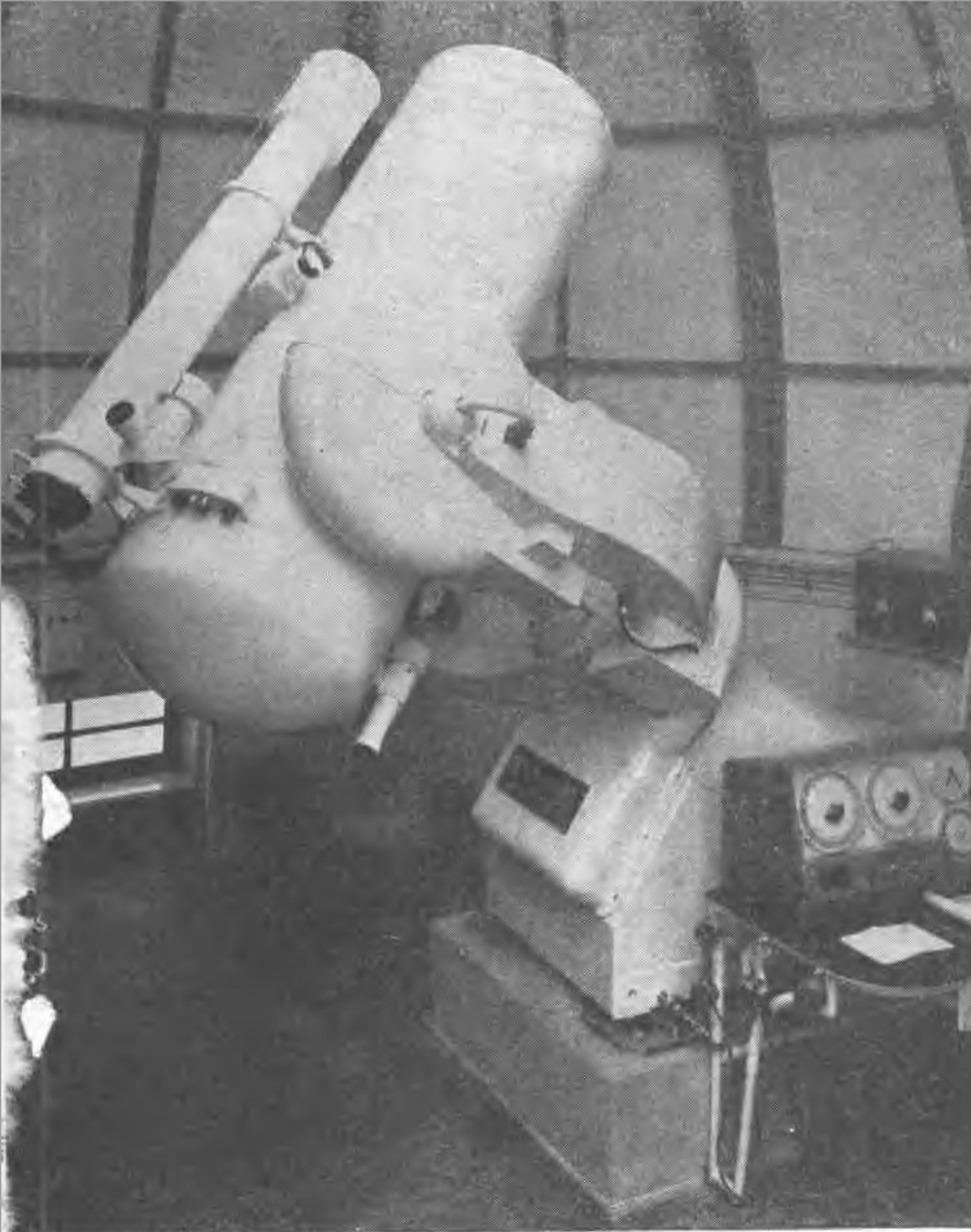
紫金山天文台 43/60/80 厘米折反射望远镜
