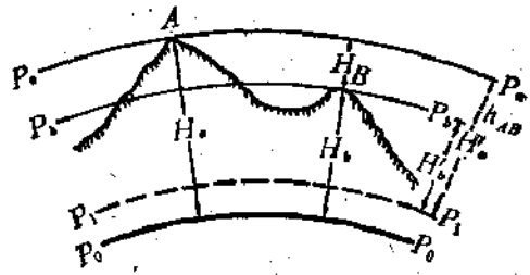
图 1-3 地面点的高程
