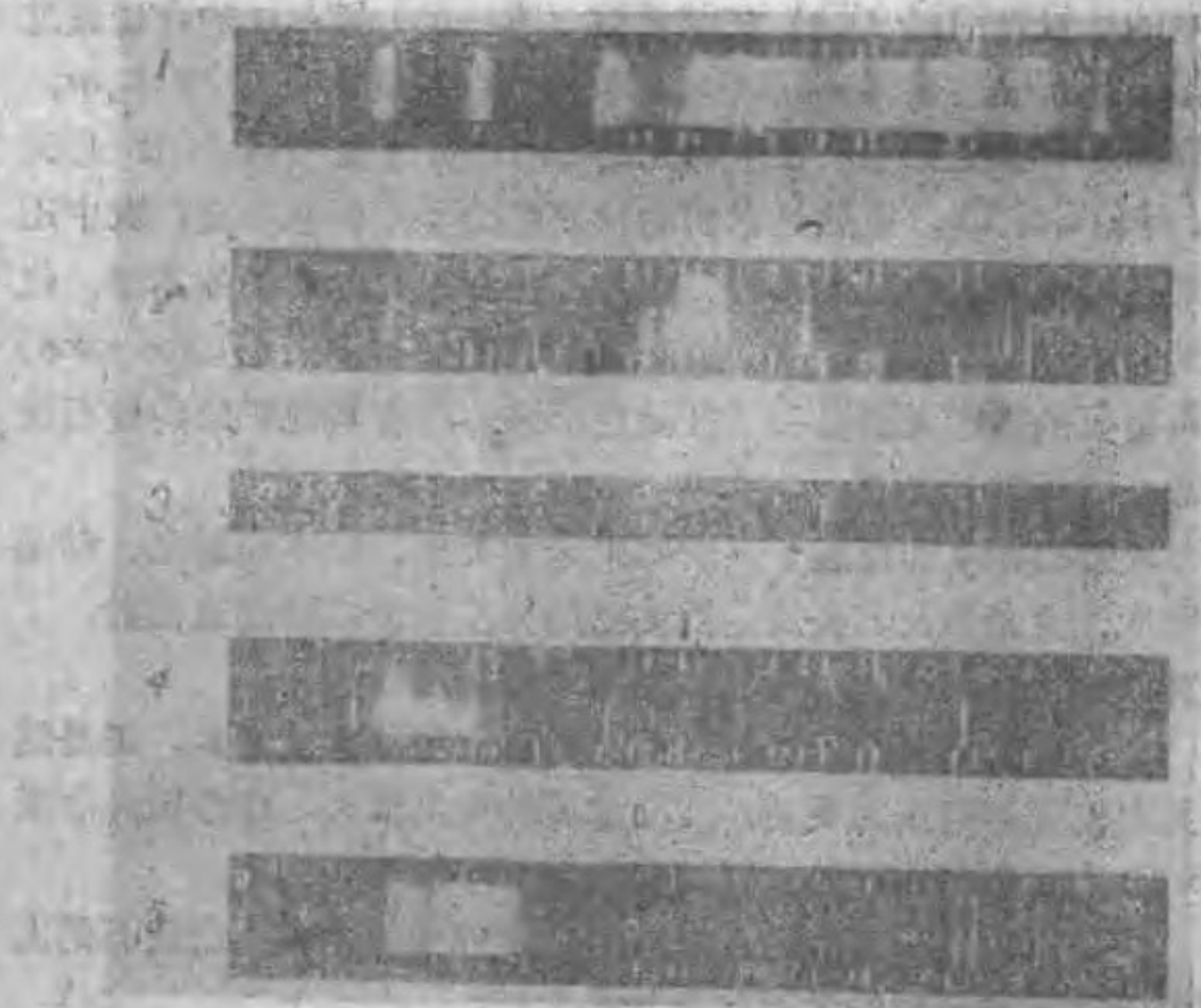
图 1. 三价离子钐 (1), 铈 (2), 钕 (3), 铕 (4), 铈 (5) 的辐射谱线
