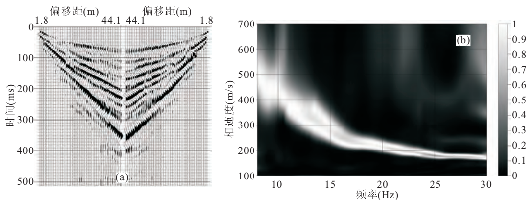
图 3 怀俄明州 SH 波的实例
