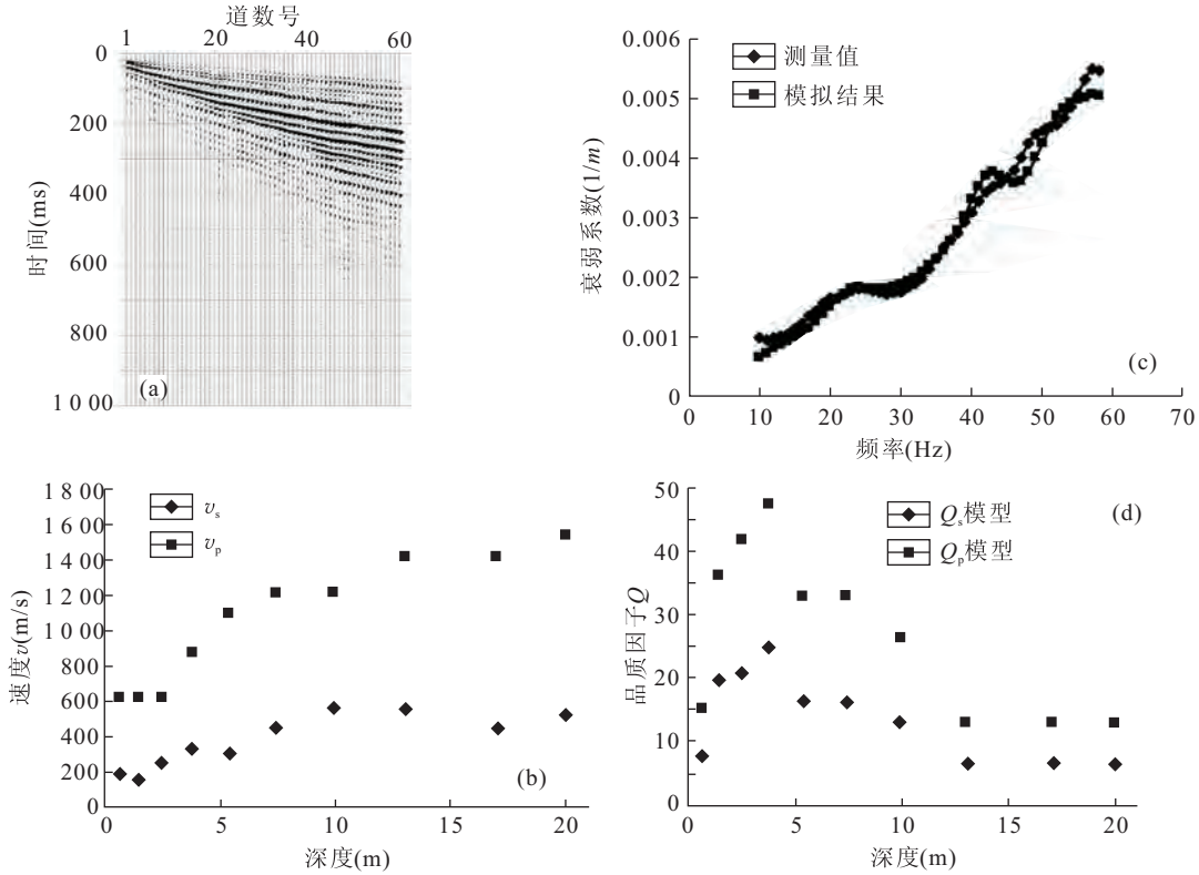
图 5 亚利桑那州沙漠的例子( Xia 等,2002)
