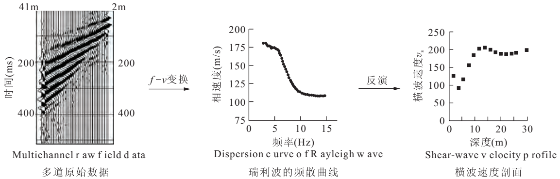
图1 面波的多道分析方法示意图
