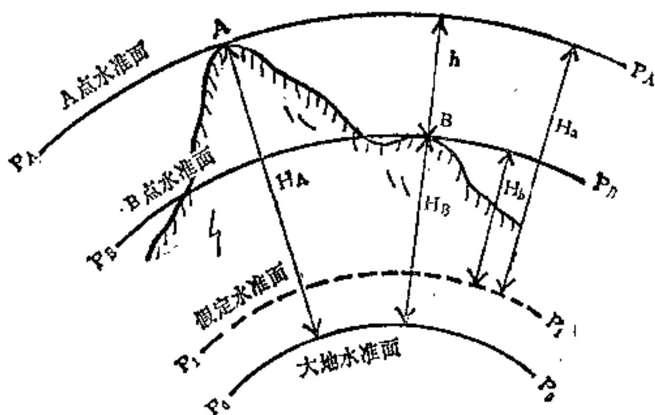
图1—4 高程
