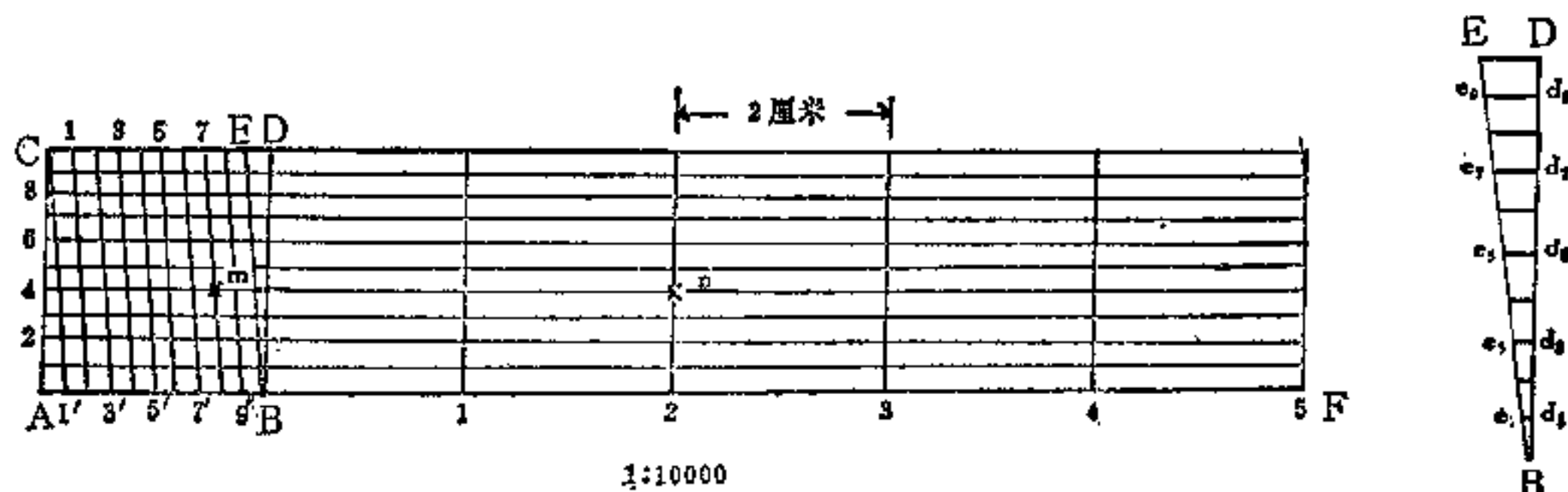
图 1—7 1:10000 复式比例尺
