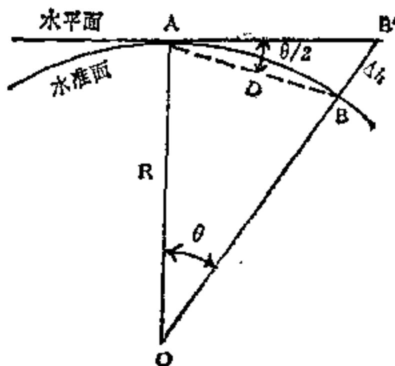
水准面作水平面的限度图
