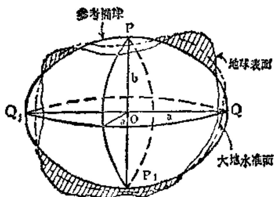
图 1—1 地球的形状
