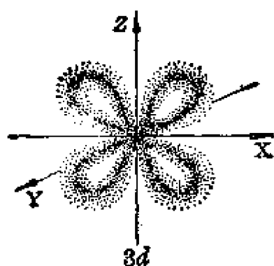
图 1-3 d 电子云
