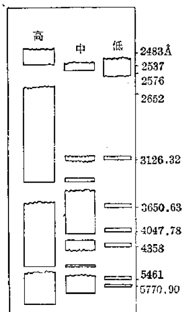
图2 高压、中压、低压汞灯发射的典型光谱
