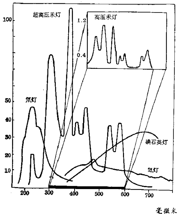
图 4 不同光源的光谱输出功率
