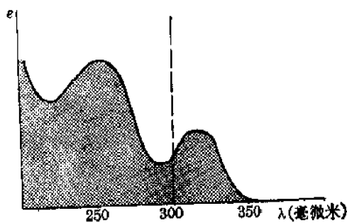
紫外吸收谱
