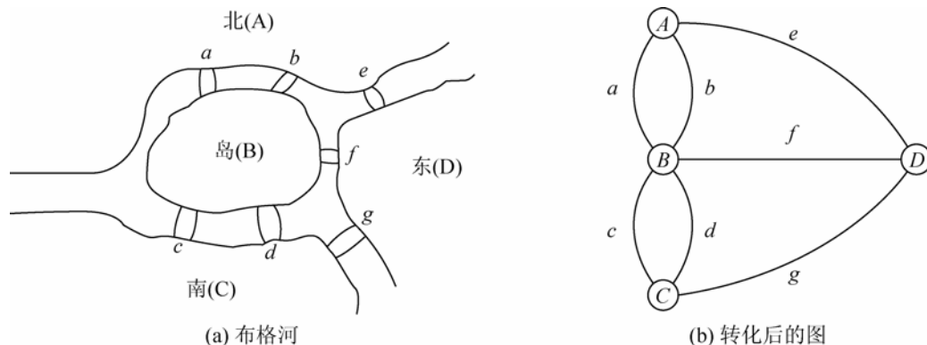
图 1 七桥问题
